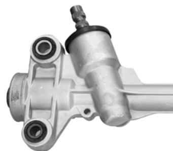
ESTRIADO 36 DIENTES
